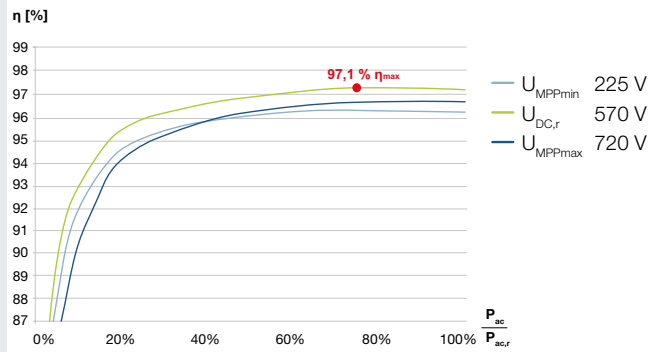
PLENTICORE plus 5.5
